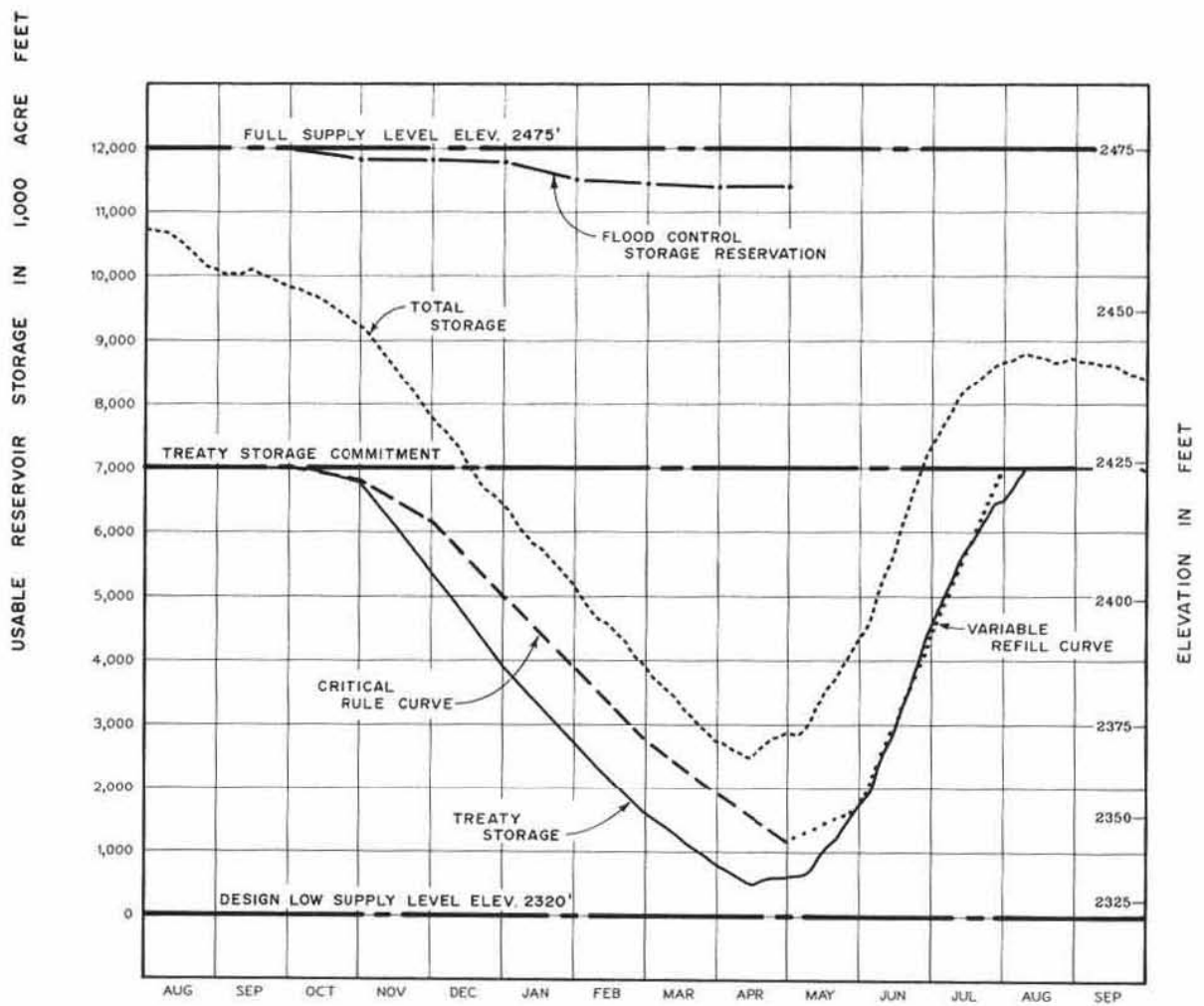
MICA RESERVOIR
